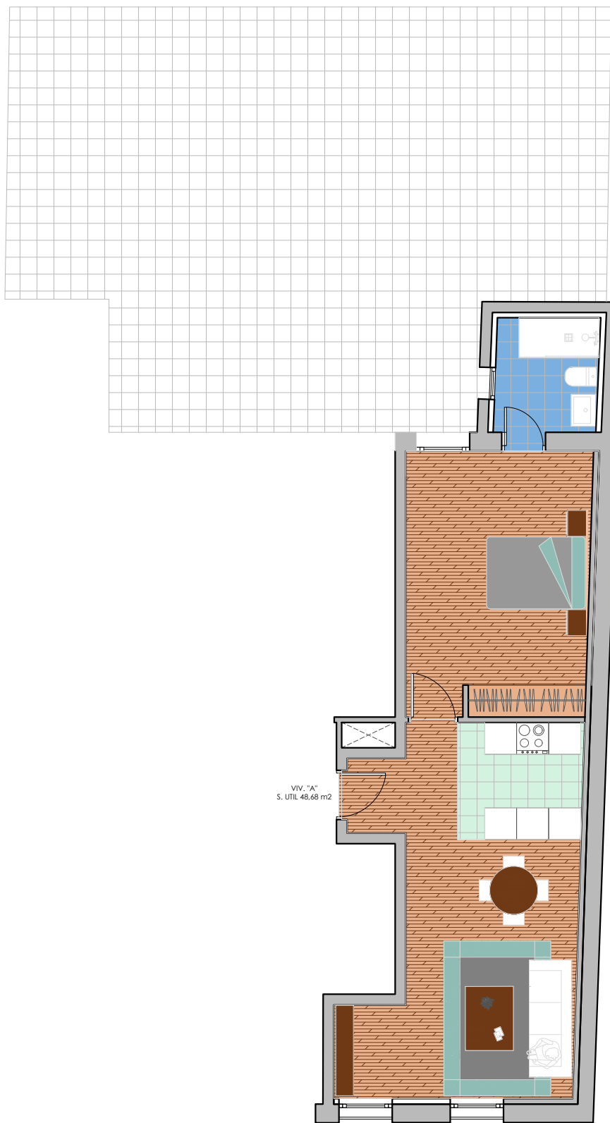
PLANTA BAJA Y ENTREPLANTA VIVIENDA A
