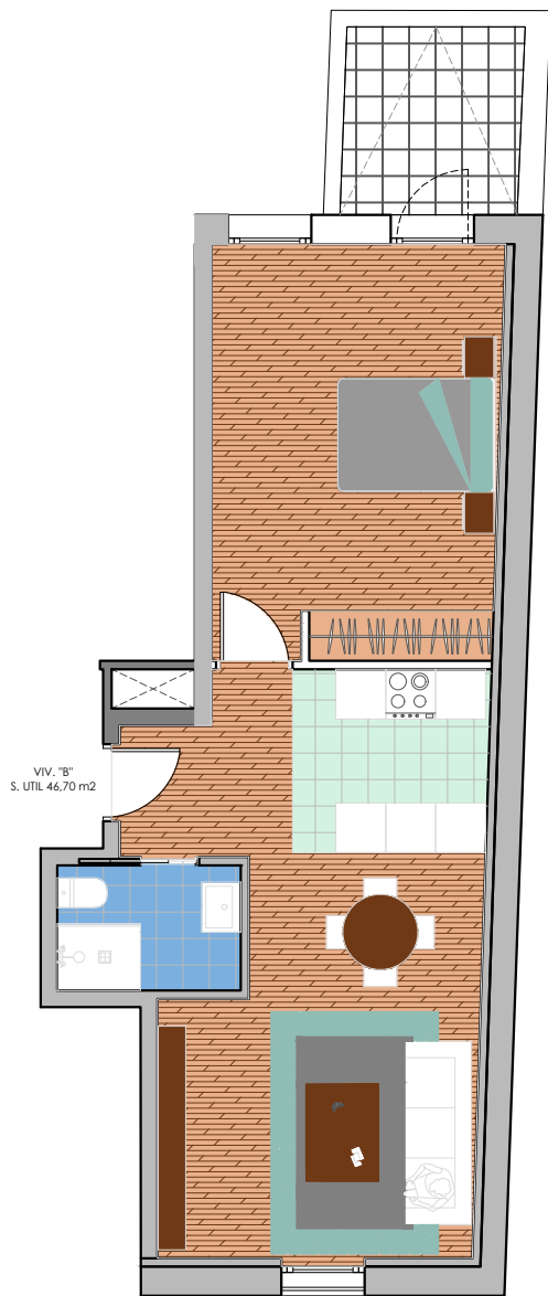
PLANTA 1 VIVIENDA B
