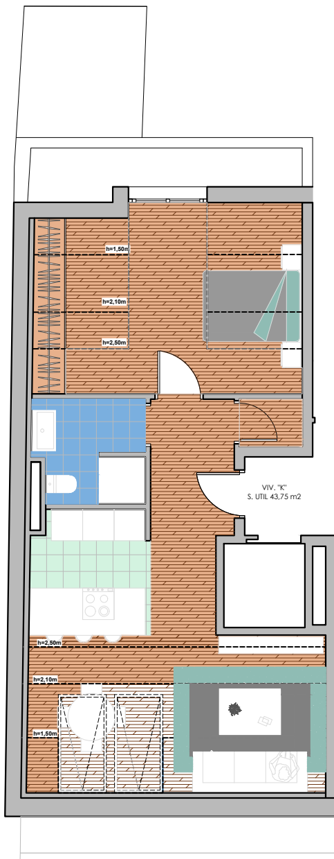
PLANTA BAJO CUBIERTA VIVIENDA K
