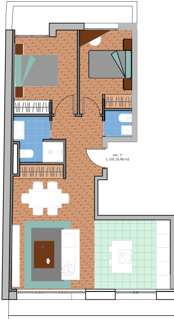
PLANTA 4 VIVIENDA I
