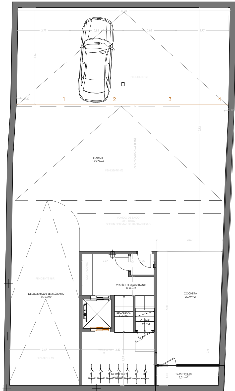
PLANTA SÓTANO Y SEMISÓTANO
